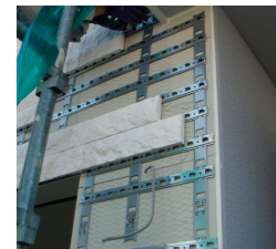
NC新シュタールネット工法
